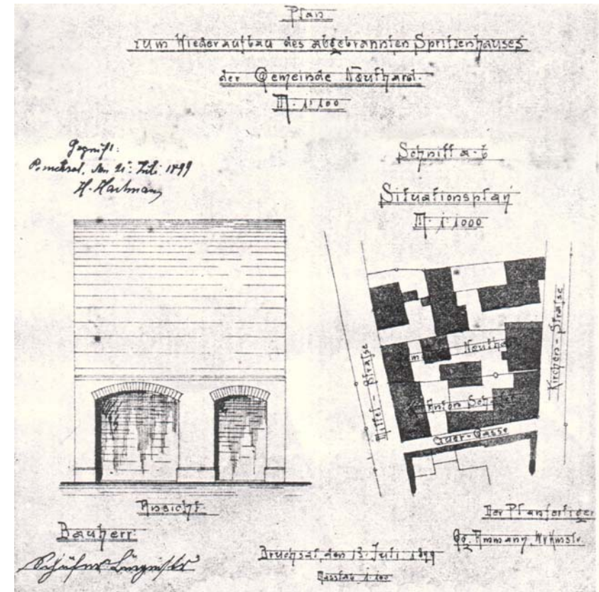
Abb. Plan des alten Spritzenhauses von 1899, ehemaliger Standort: Verbindung Volksbank/Apotheke
